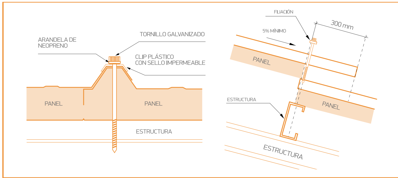
TRANSVERSAL
