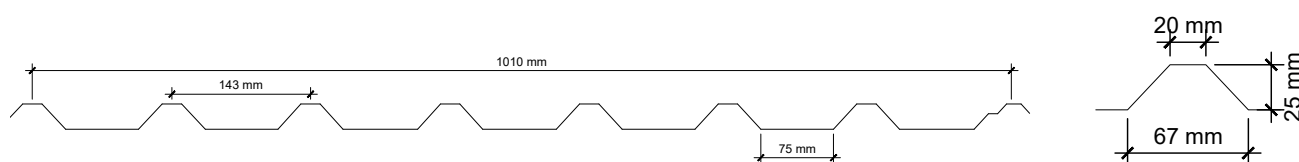
Perfil de lámina troquelada D-101
